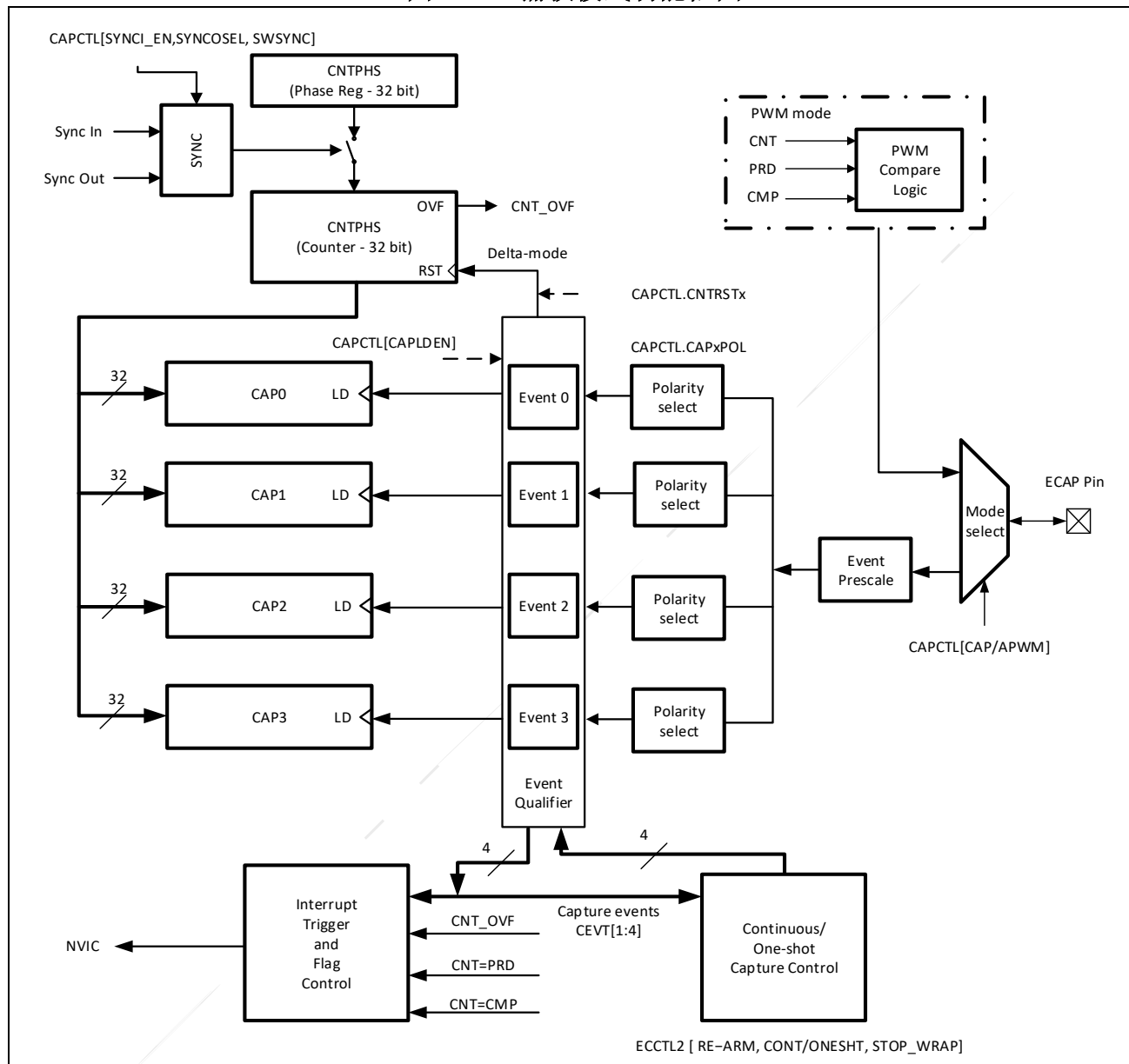
图 11-3：捕获模式功能框图
