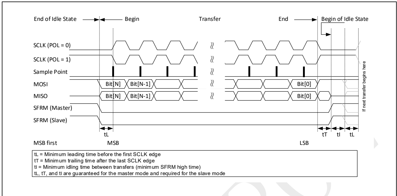
图 19-4: SSP 时钟格式 0 (PHS = 0)
