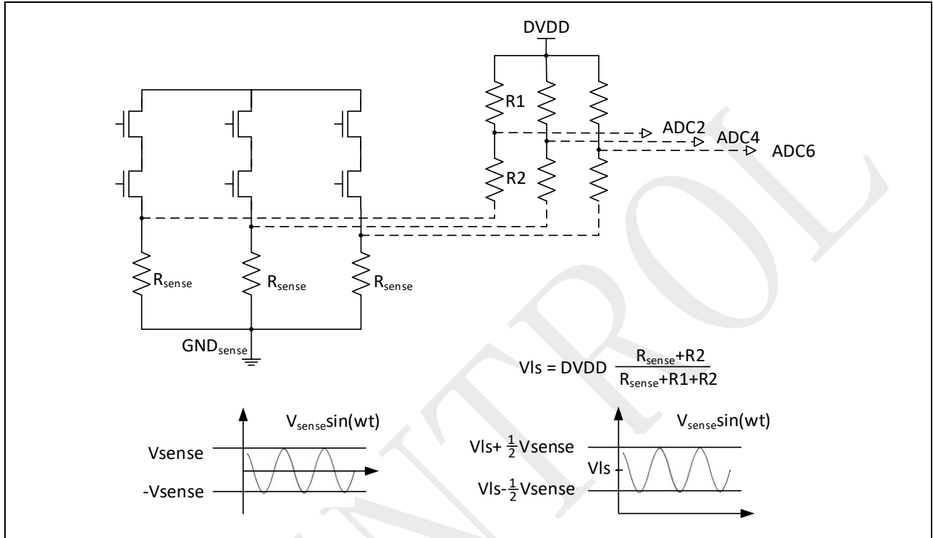
图 14-4：PGA0 选择 ADC4 作为输入（单端模式）
