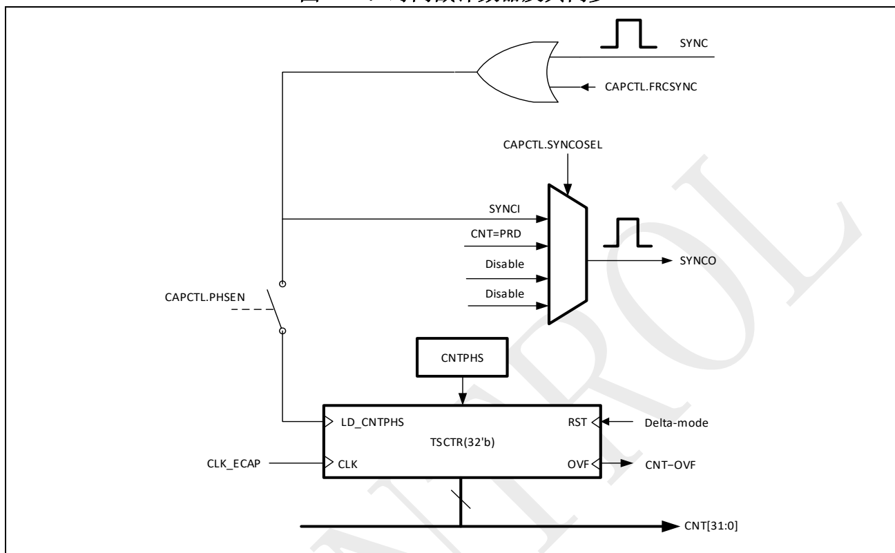
图 11-7：时间戳计数器及其同步
