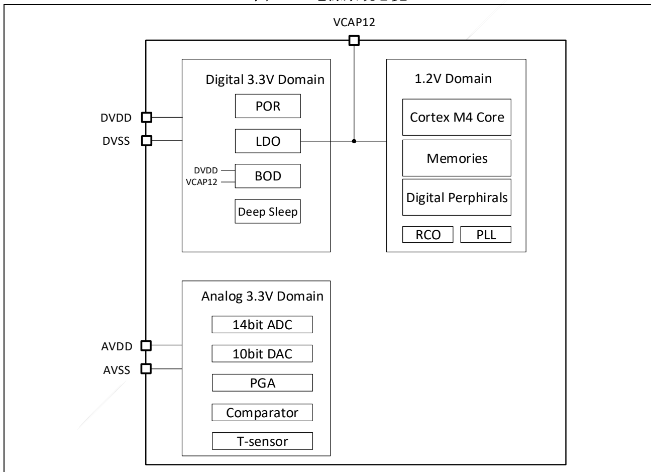
图 2-1：电源系统总览
