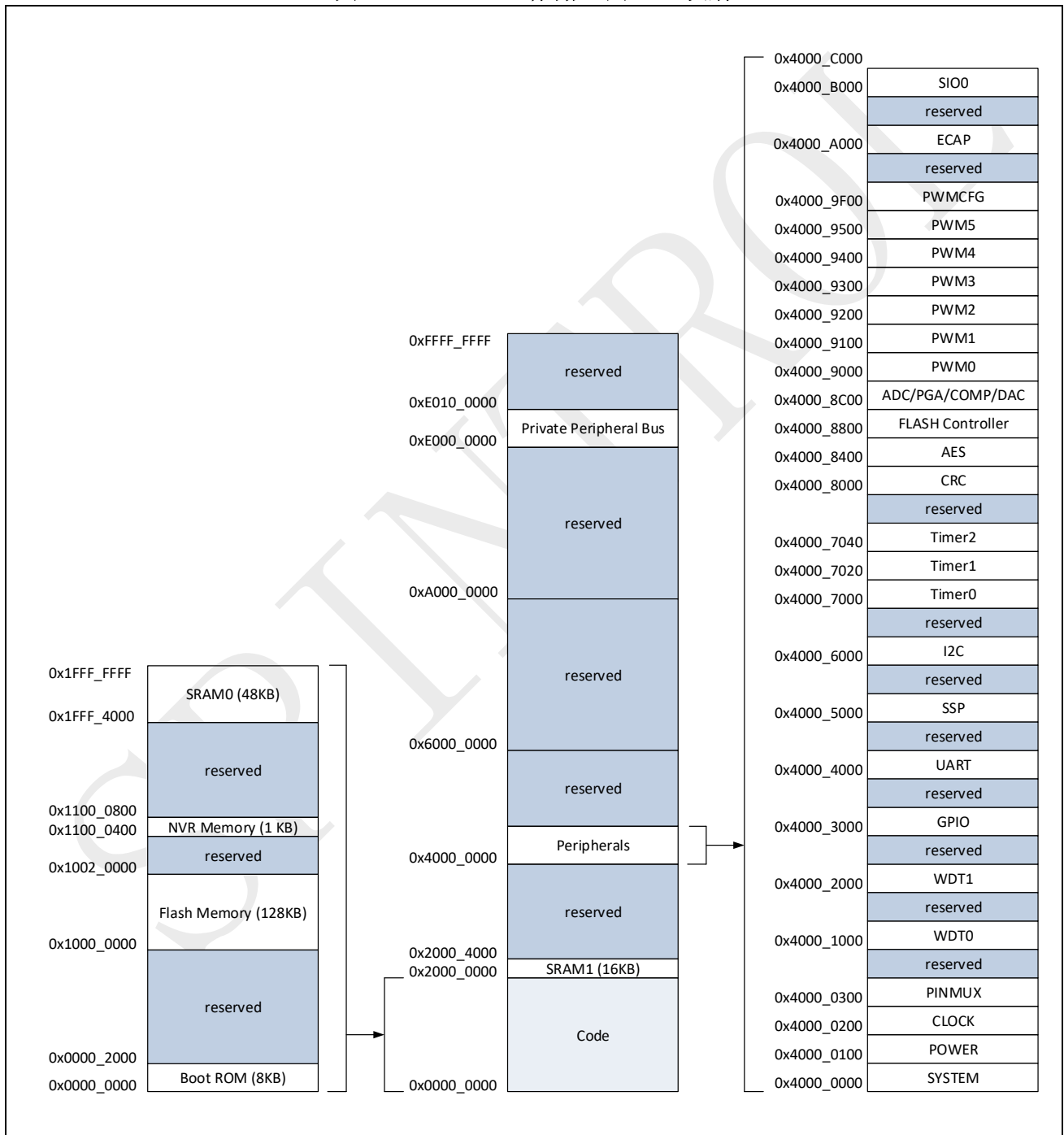
图 1-3：SPC1168 存储空间地址映射
