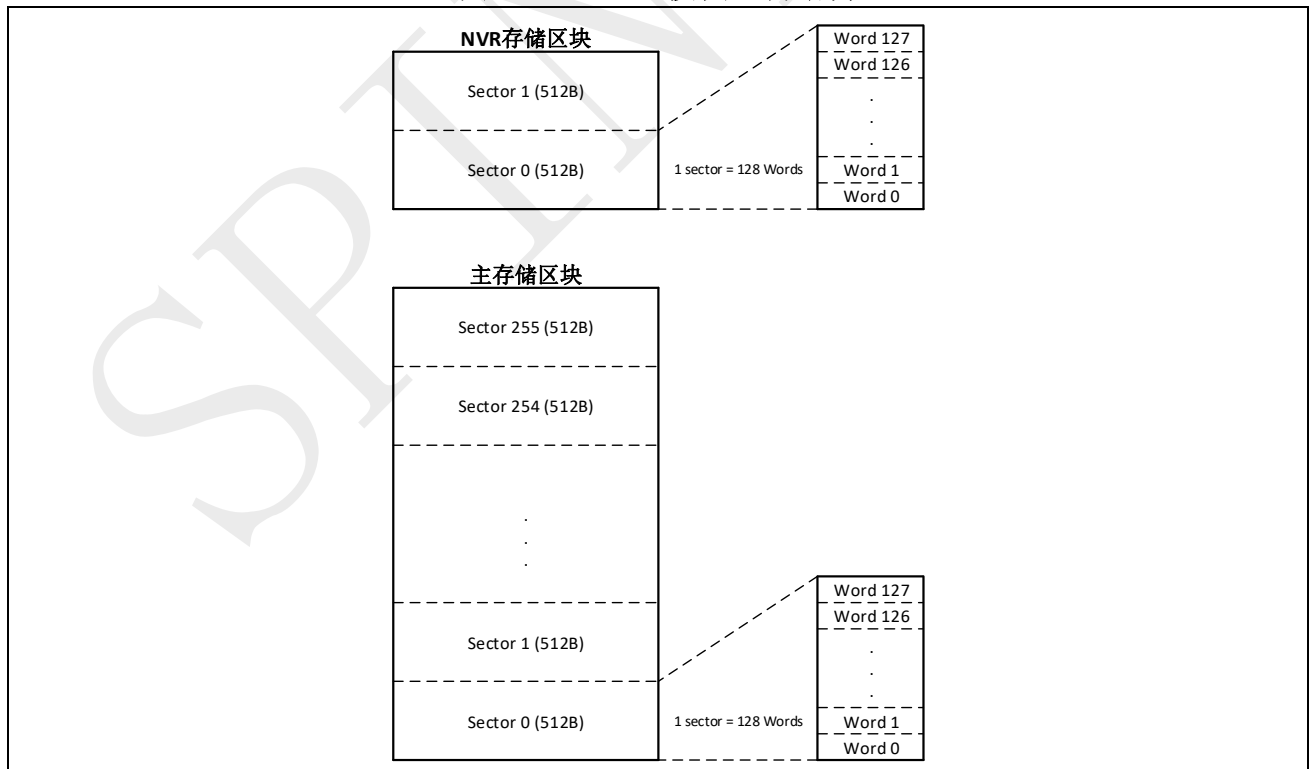
图 20-2: Flash 模块逻辑结构
