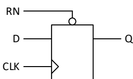
带异步复位的D触发器
