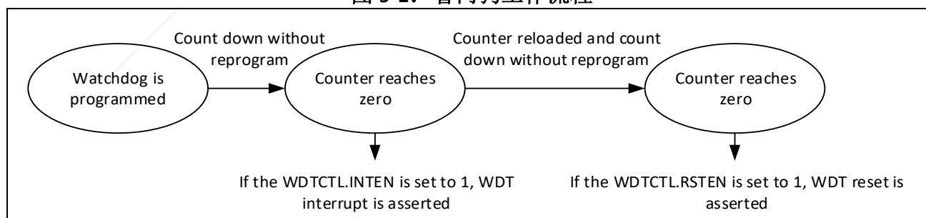
图 9-1：看门狗工作流程
