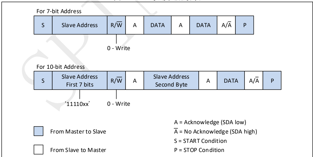
图 18-5：主机-发送器协议
