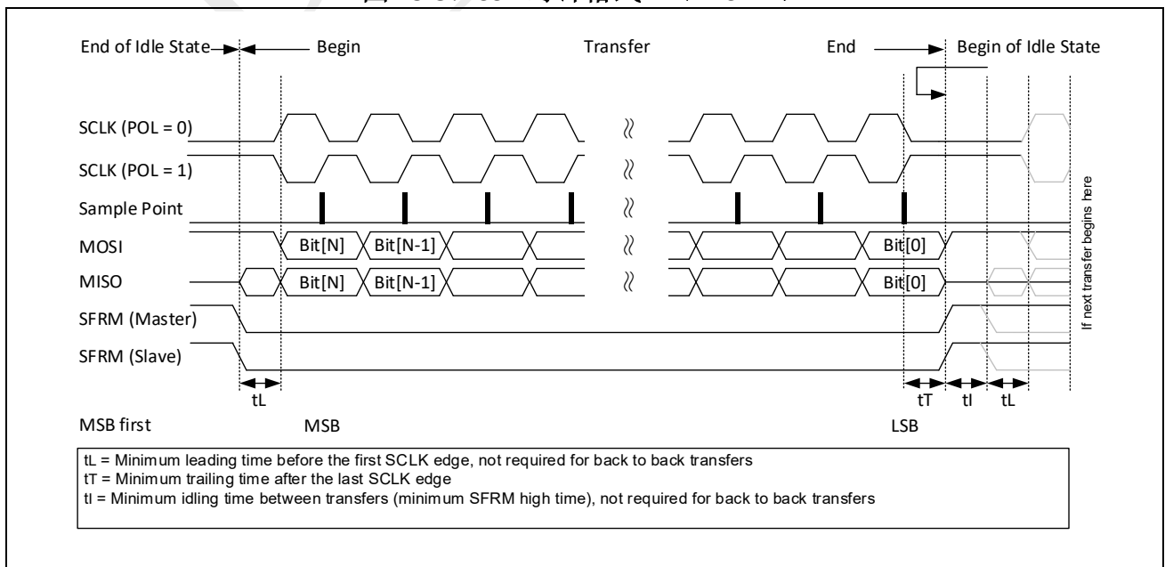
图 19-5: SSP 时钟格式 1 (PHS = 1)
