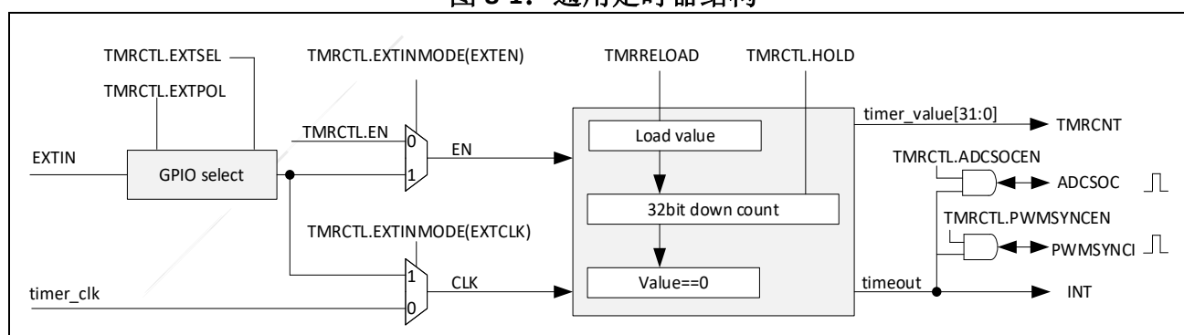
图 8-1：通用定时器结构
