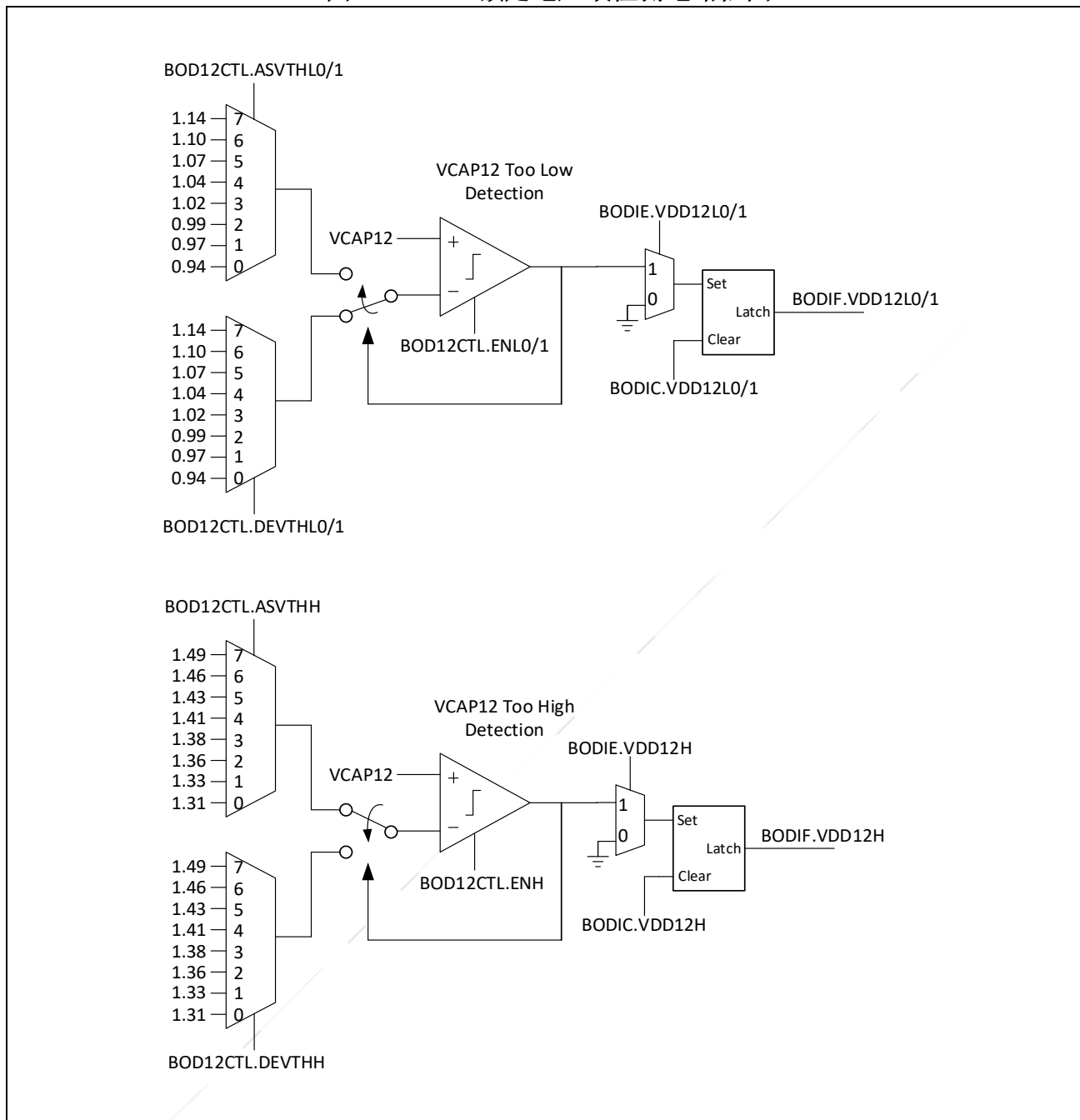
图 2-3: 1.2V 额定电压域检测电路框图
