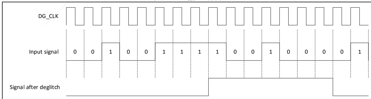
图 4-4：输入消抖
