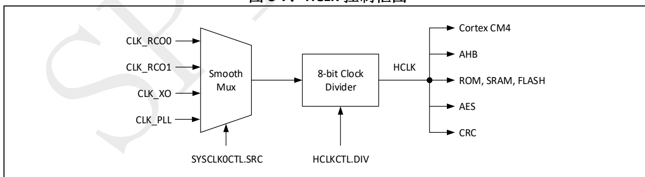
图 3-7: HCLK 控制框图
