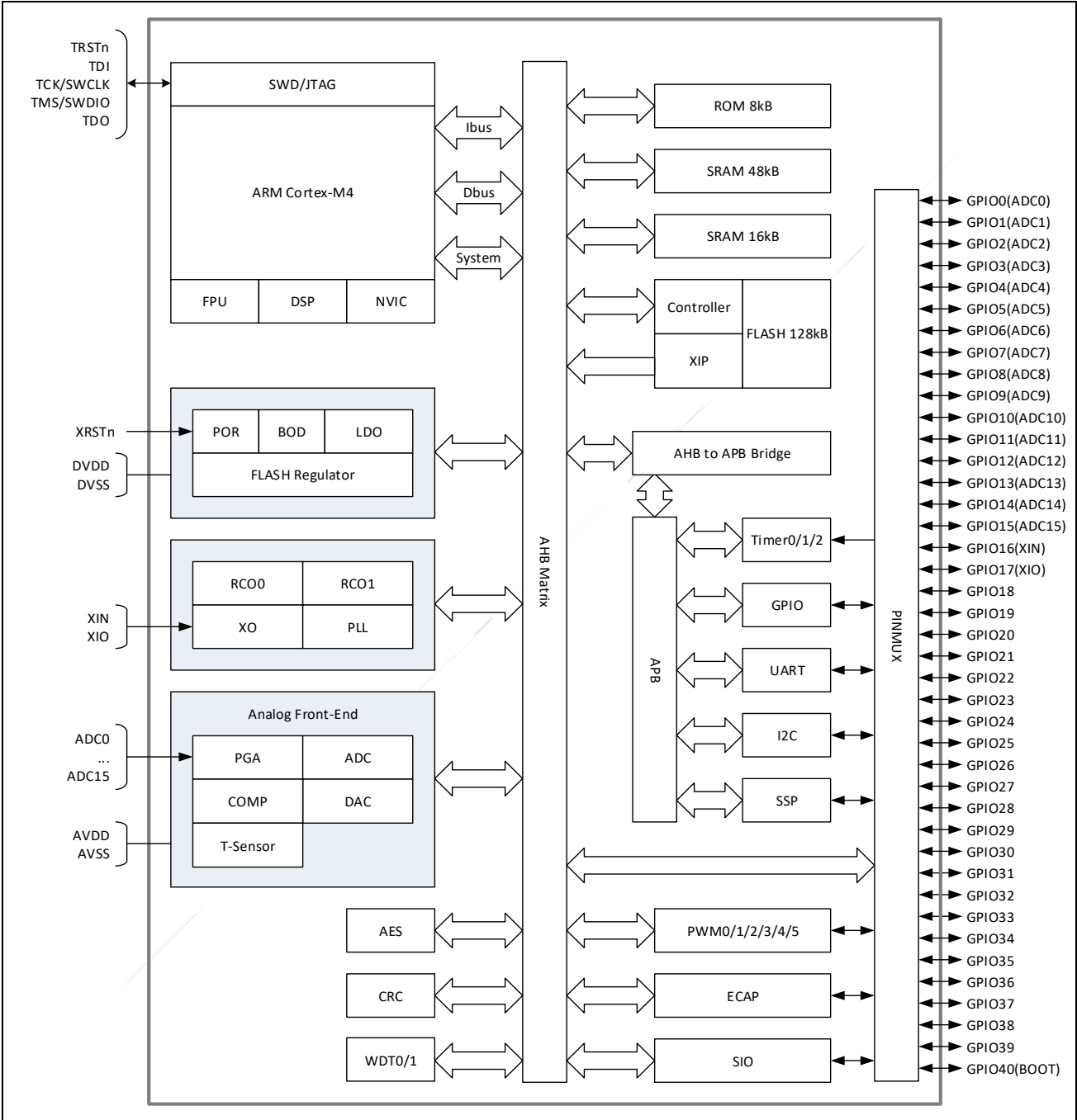
图 1-1: SPC1168 系统框图
