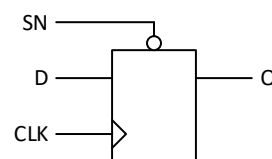
带异步置位的D触发器
