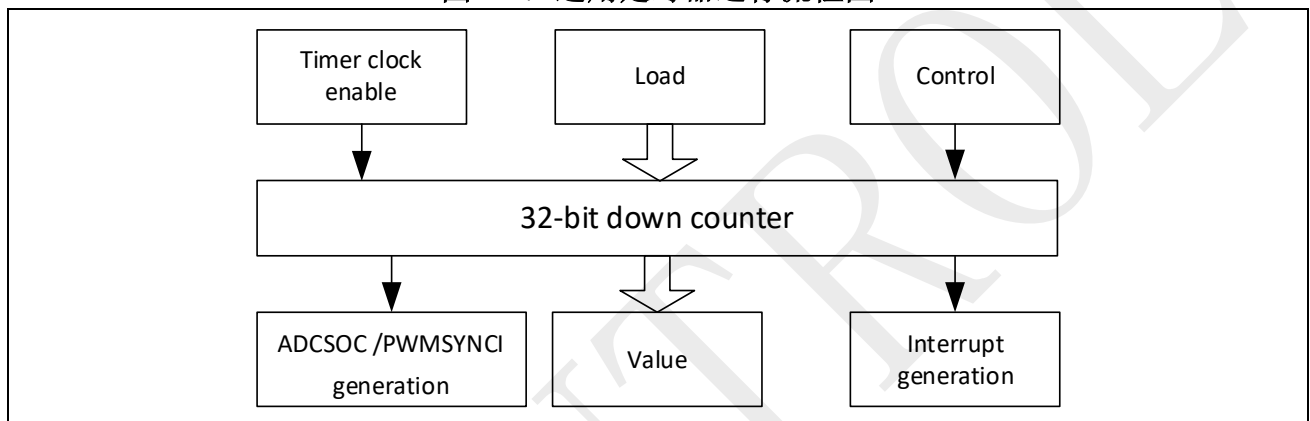
图 8-2：通用定时器运行流程图
