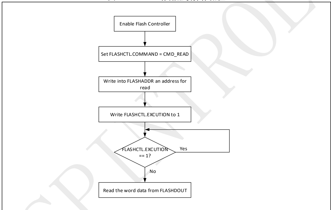
图 20-3: Flash 存储器读操作流程
