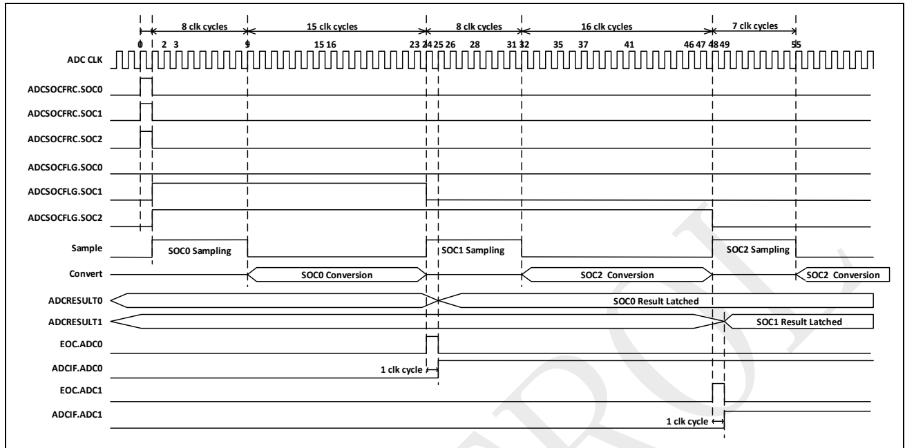
图 12-13: 同时采样模式时序
