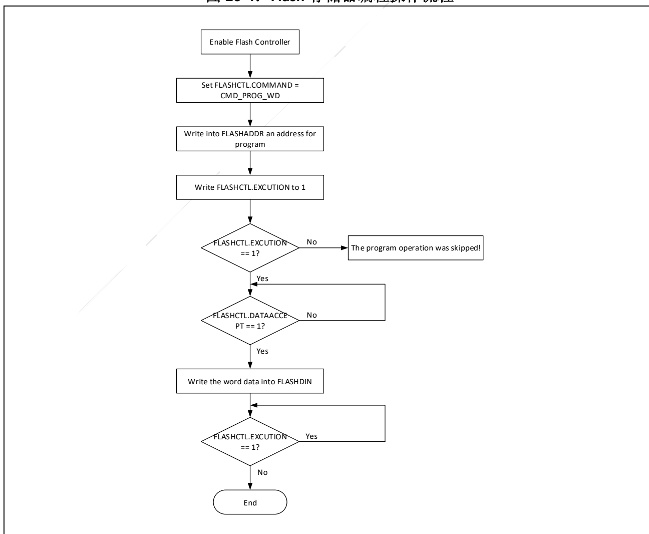
图 20-4: Flash 存储器编程操作流程
