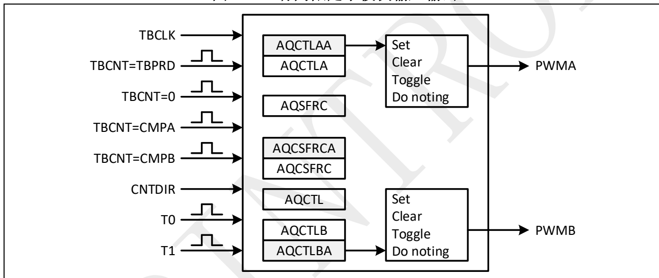
图 10-8：行为限定子模块输入输出
