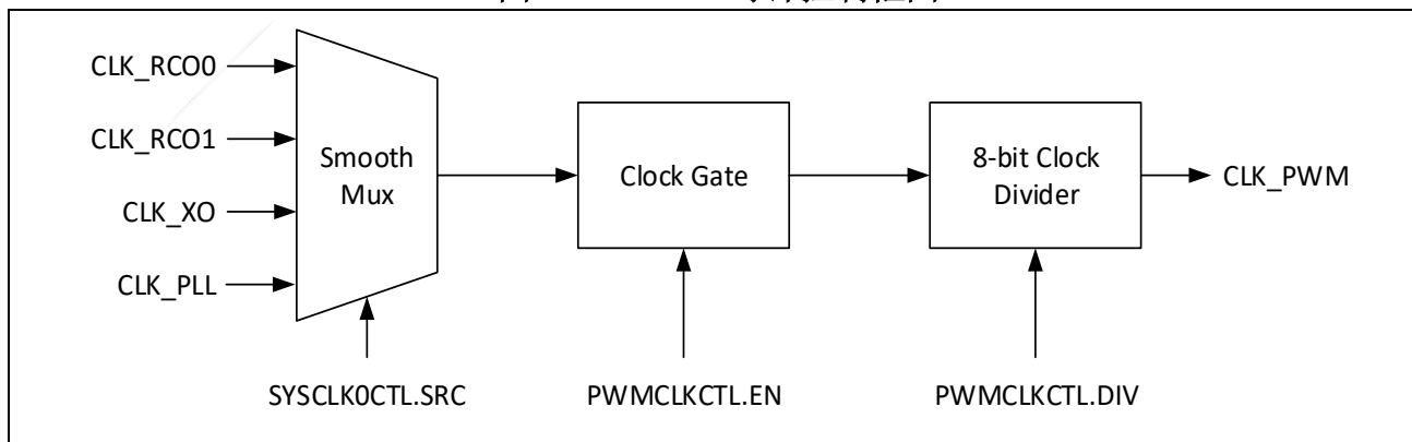
图 3-14：PWM 时钟控制框图
