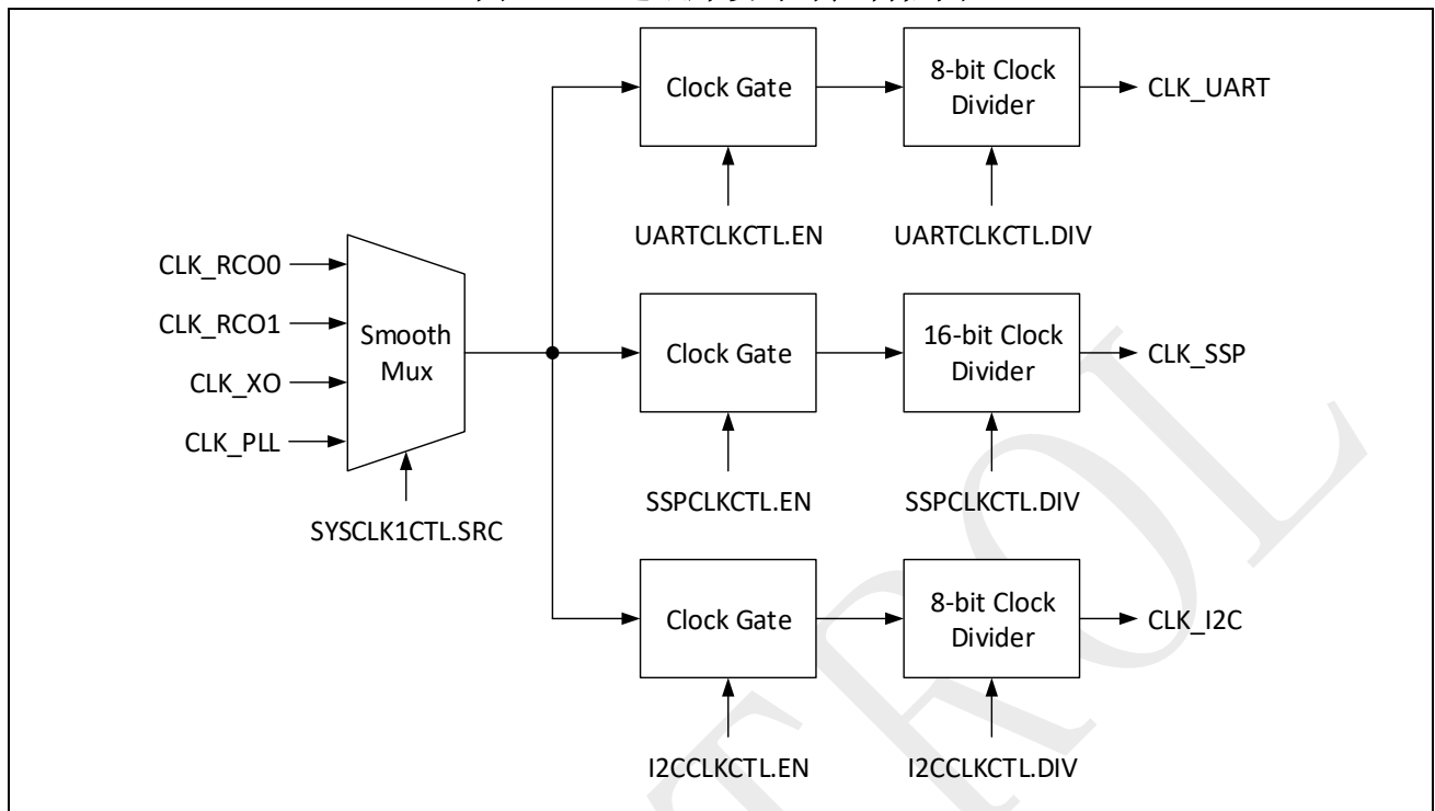
图 3-10: 通讯外设时钟控制框图
