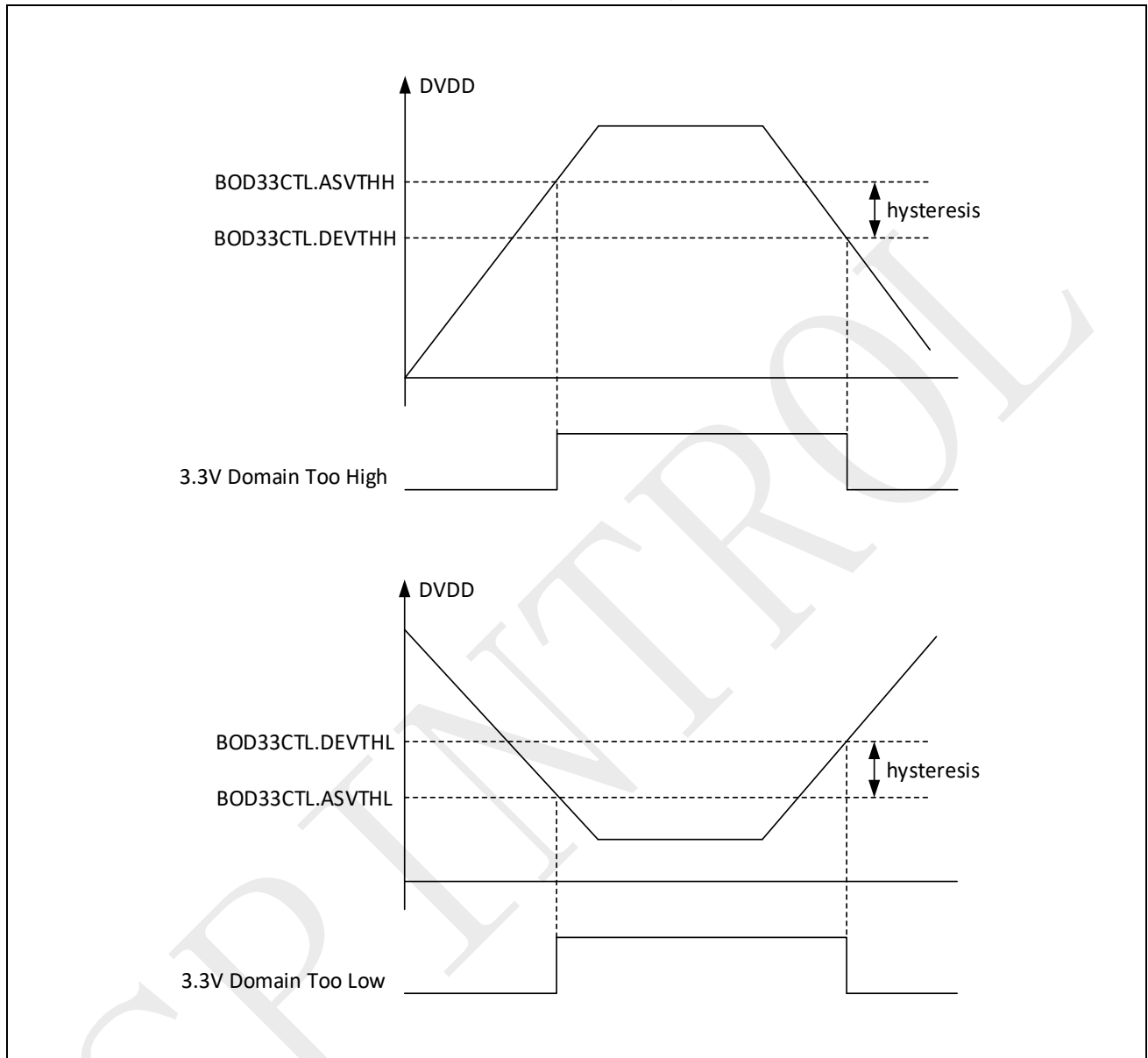
图 2-4: DVDD 阈值
