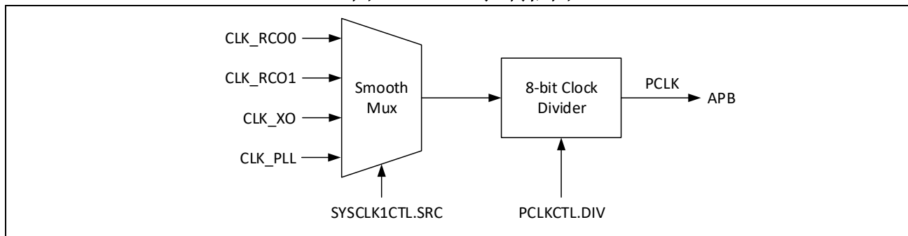
图 3-8: PCLK 控制框图
