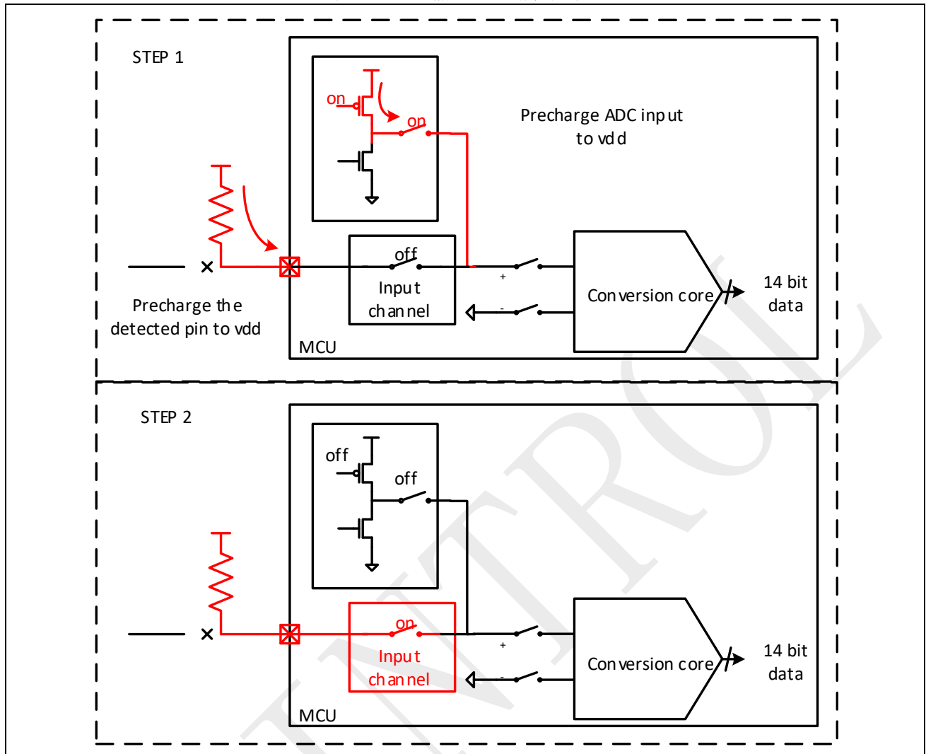
图 12-17: 检测 ADC 输入 PIN 脚断路 (预充电)
