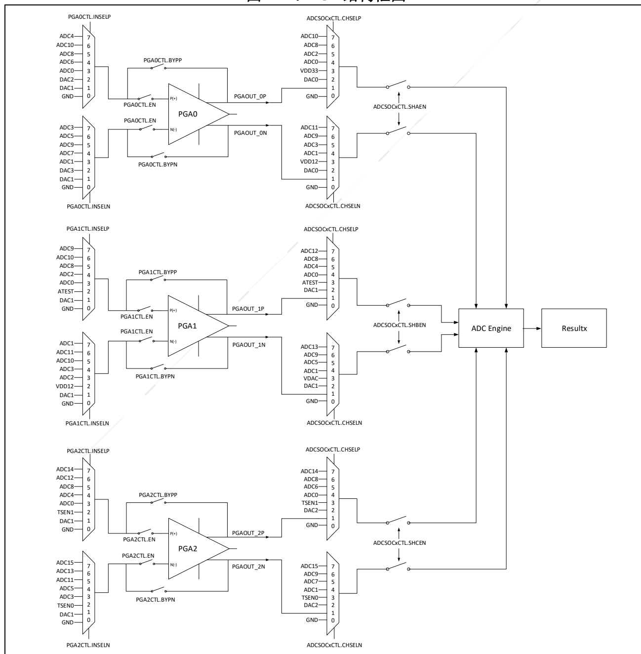
图 14-1: PGA 结构框图
