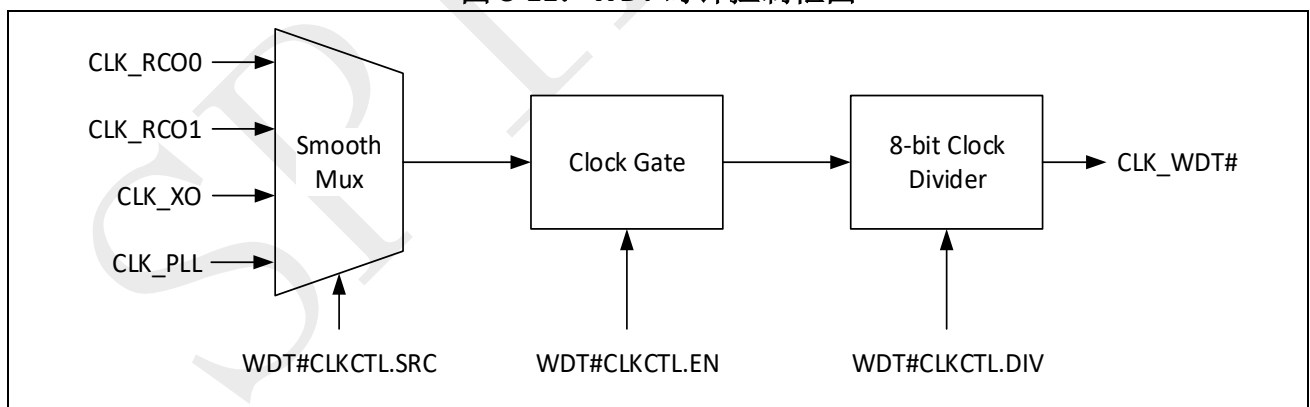
图 3-11: WDT 时钟控制框图
