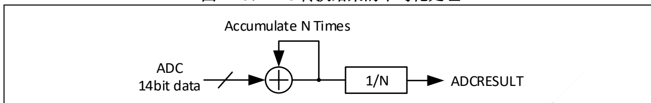
图 12-5: ADC 转换结果的平均化处理
