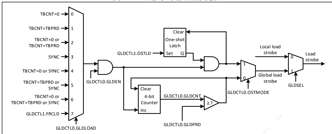
图 10-21: 影子寄存器全局读入
