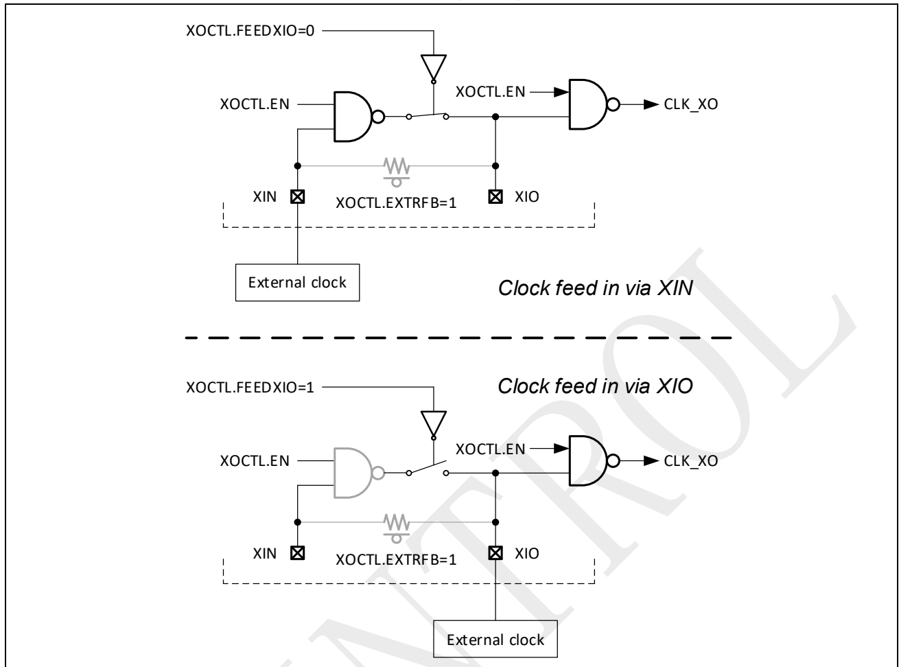
图 3-4: 外部时钟模式
