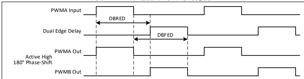
图 10-13: 双边沿延迟死区控制波形
