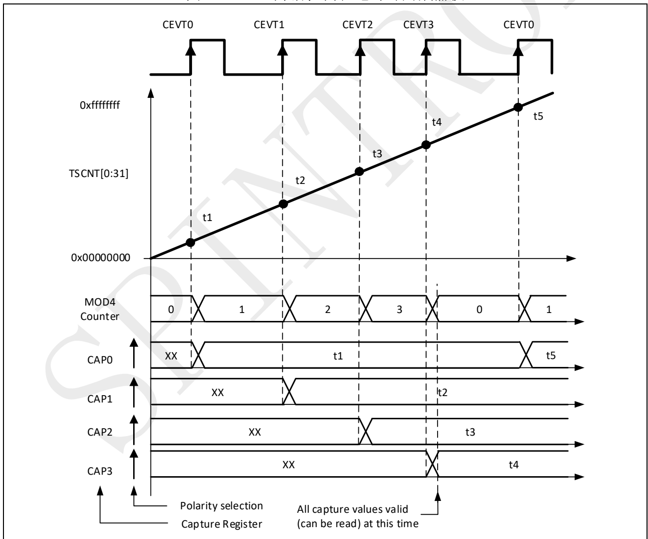
图 11-11：上升沿检测和绝对时间戳捕获
