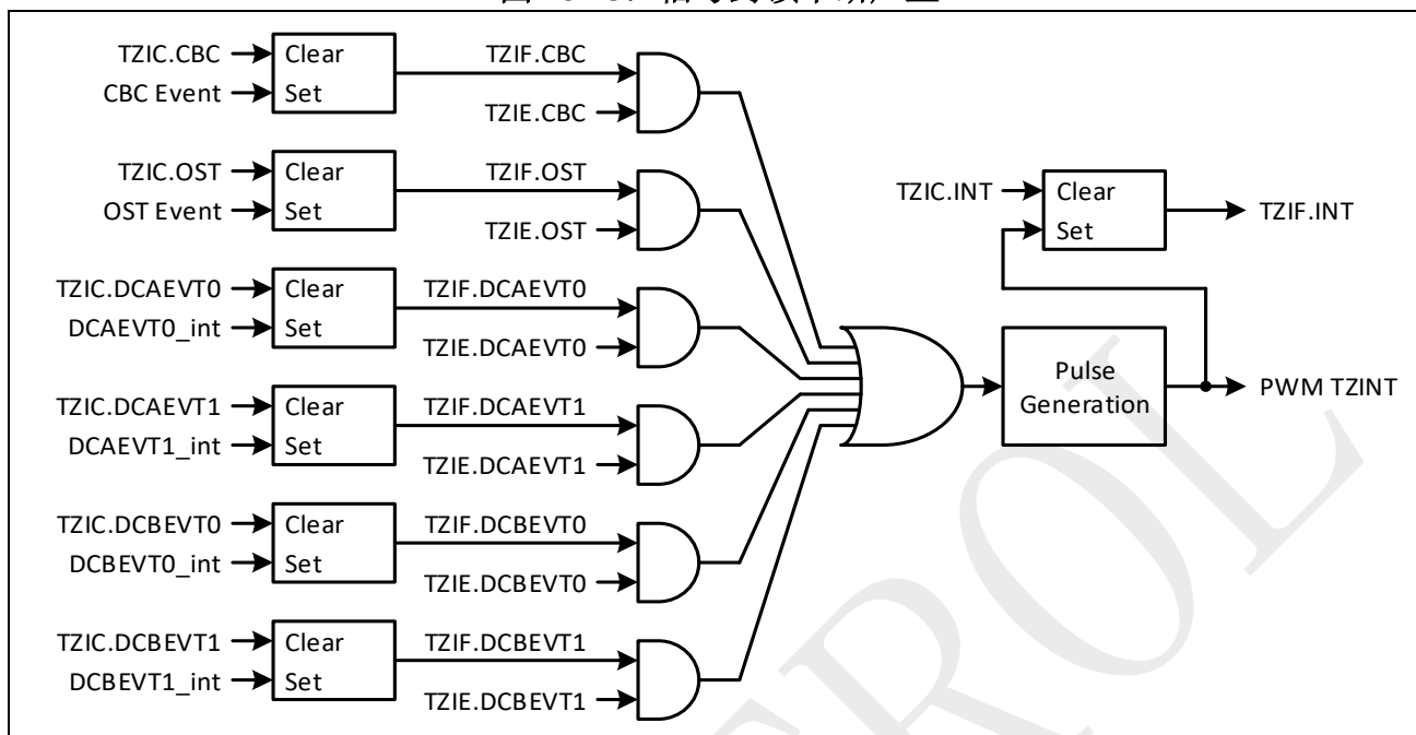
图 10-15: 信号封锁中断产生
