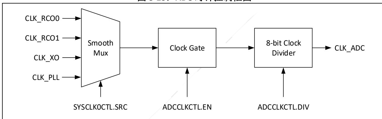
图 3-13：ADC 时钟控制框图
