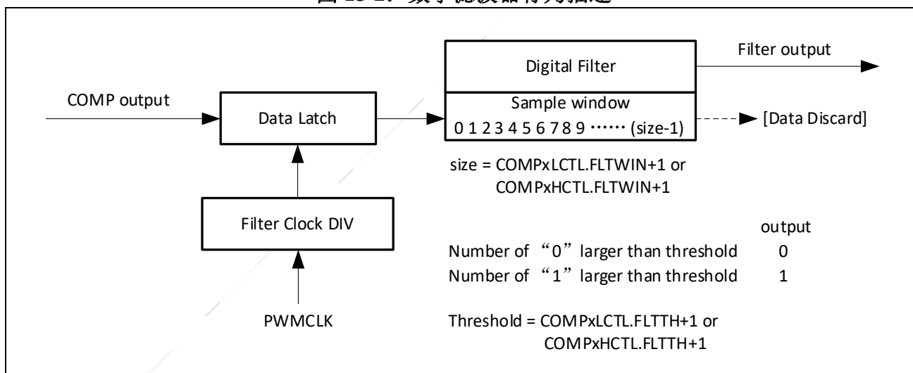
图 15-2：数字滤波器行为描述
