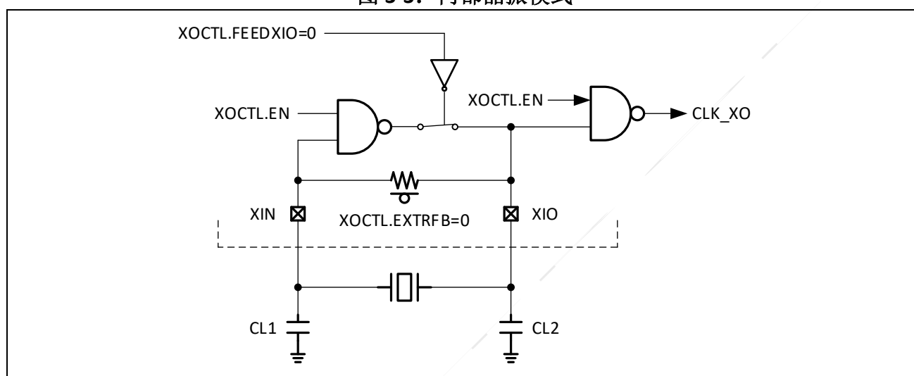
图 3-3：内部晶振模式
