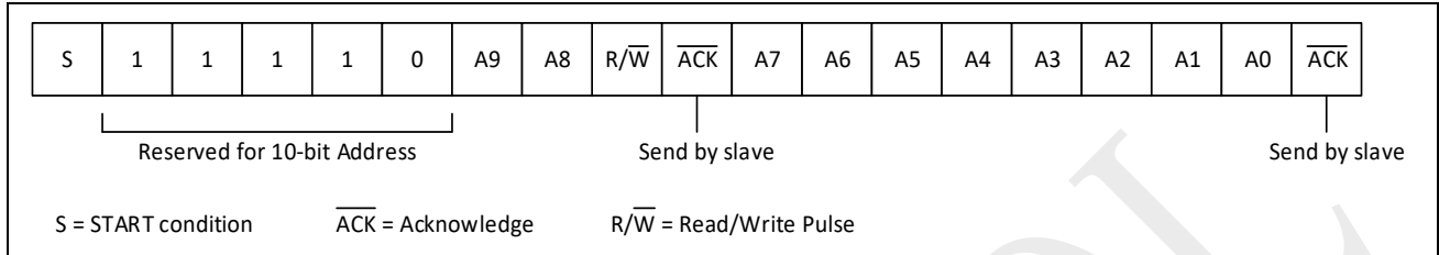
图 18-4：10 位地址格式
