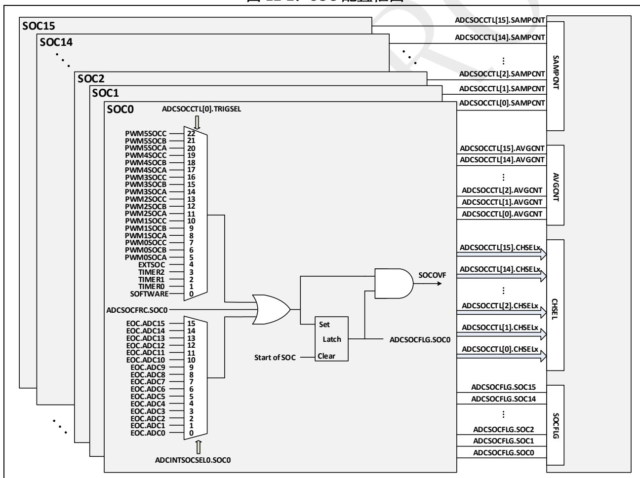
图 12-2: SOC 配置框图
