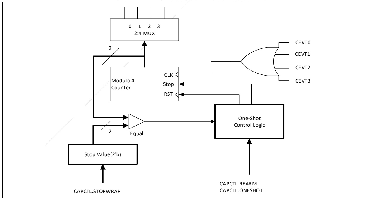
图 11-6：持续捕获和一次性捕获逻辑
