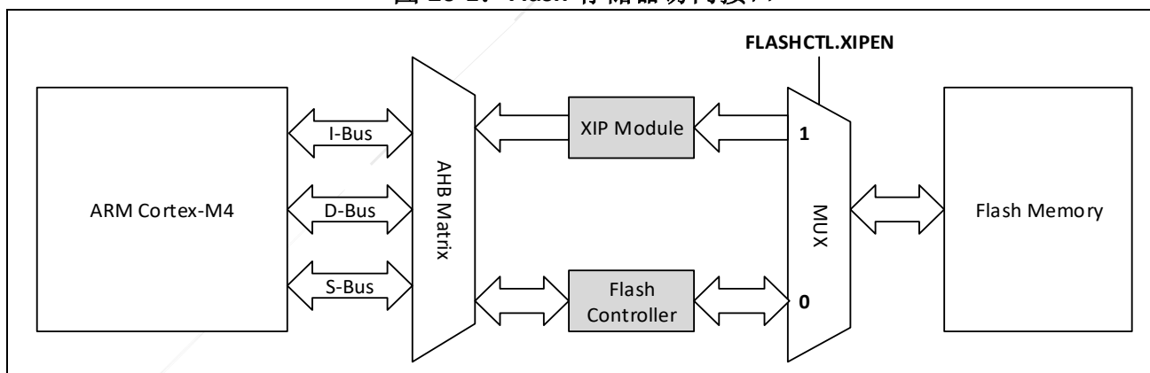
图 20-1: Flash 存储器访问接口
