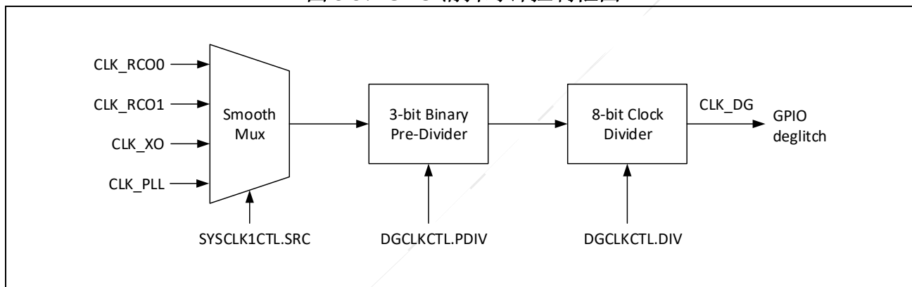
图 3-9: GPIO 消抖时钟控制框图
