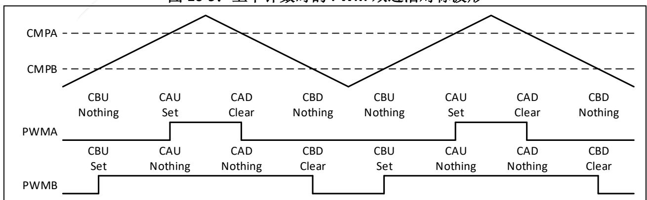
图 10-9：上下计数时的 PWM 双边沿对称波形
