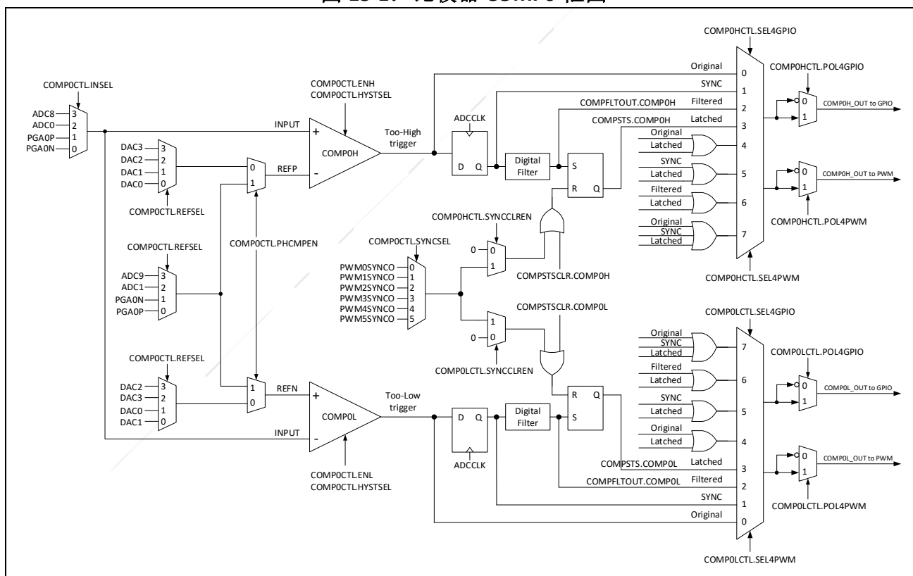
图 15-1: 比较器 COMP0 框图
