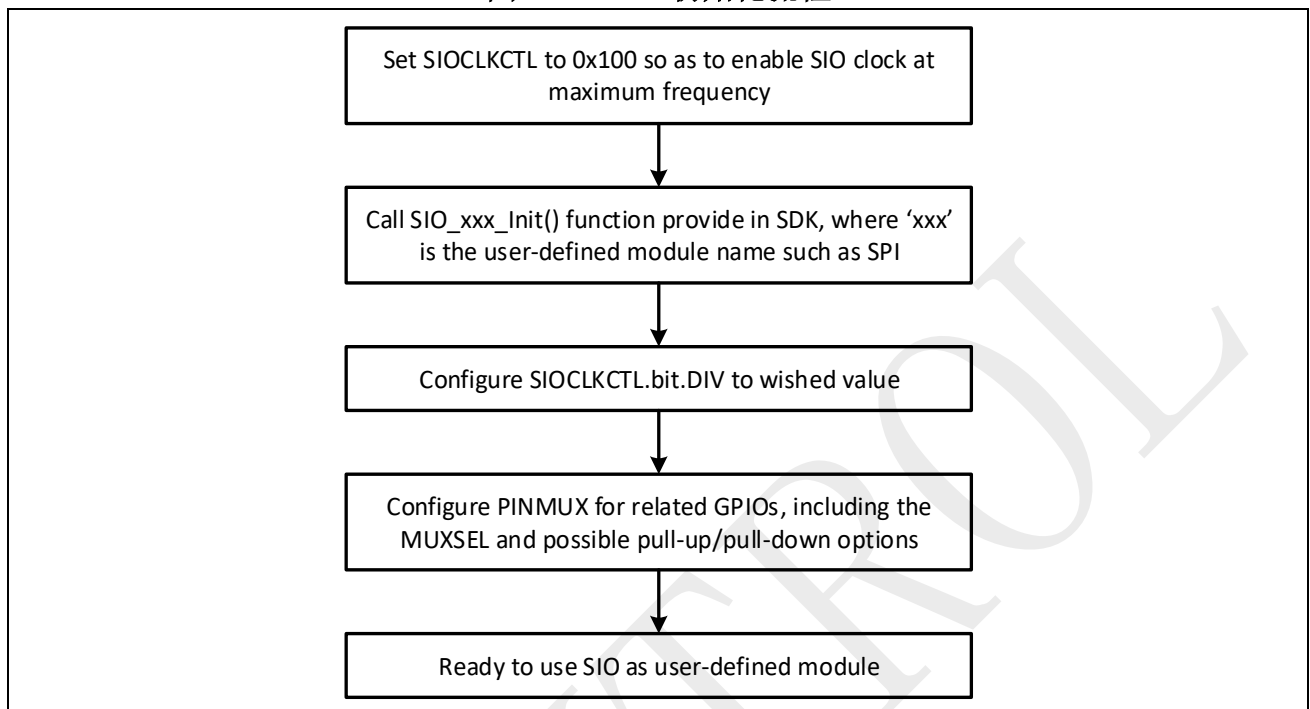
图 21-2: SIO 初始化流程
