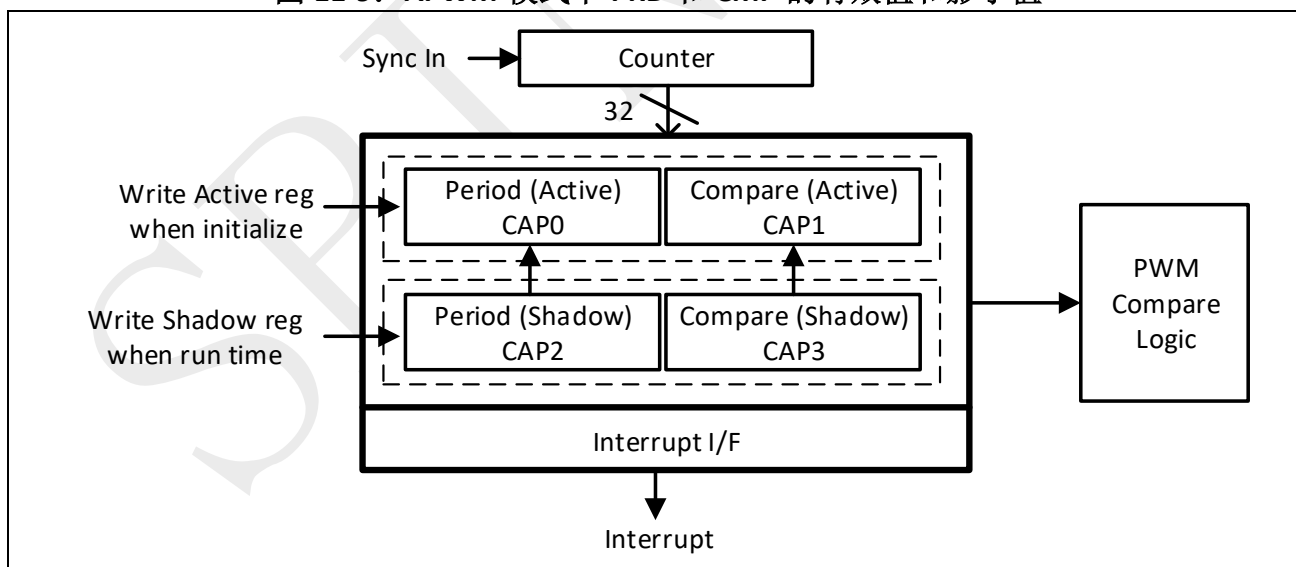
图 11-9：APWM 模式下 PRD 和 CMP 的有效值和影子值
