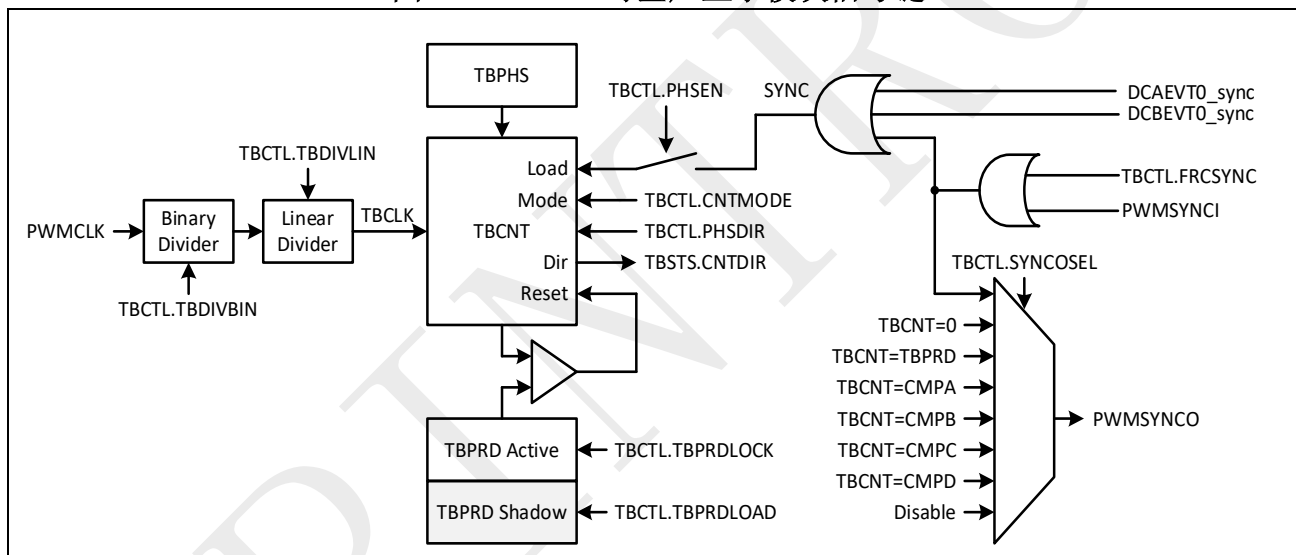
图 10-3: PWM 时基产生子模块信号链
