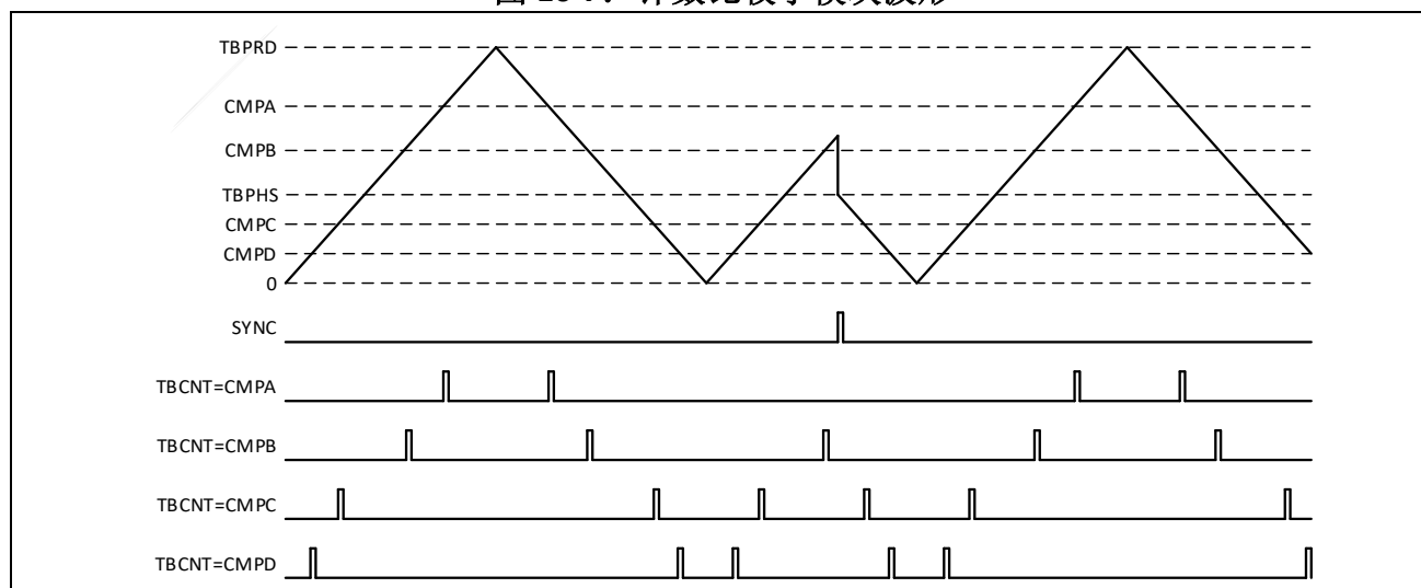
图 10-7：计数比较子模块波形
