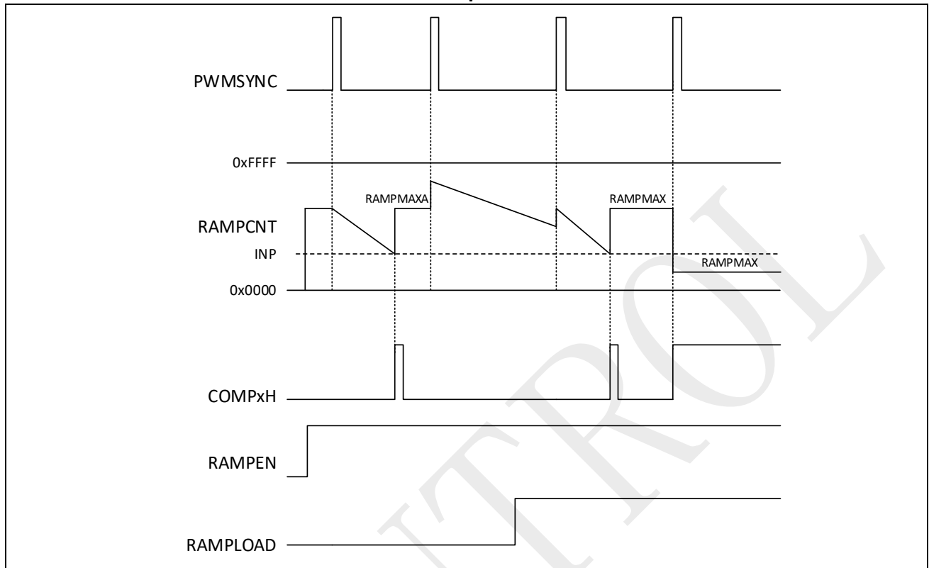
图 16-3: Ramp 发生器波形
