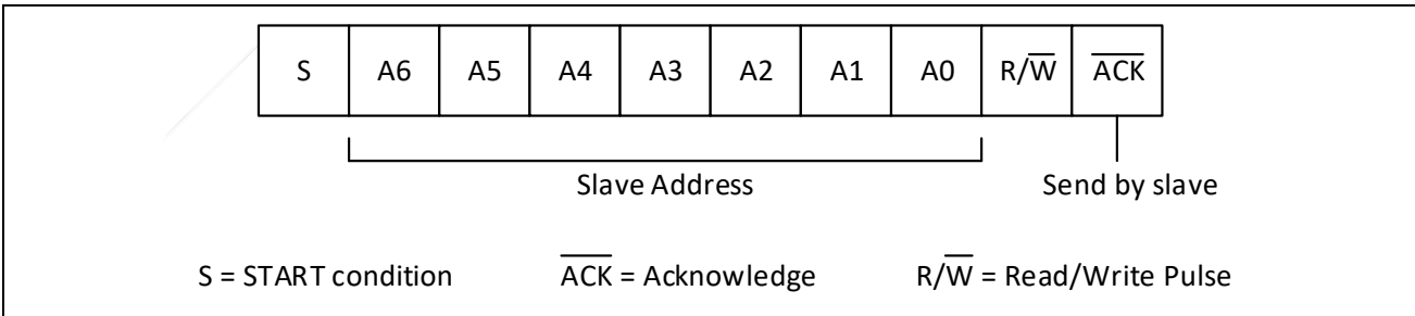
图 18-3: 7 位地址格式
