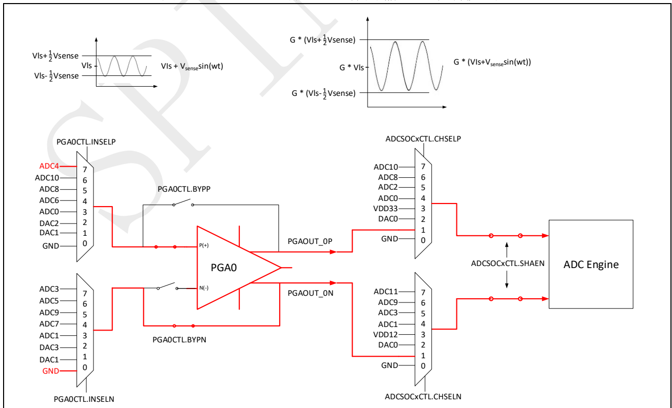
图 14-4：PGA0 选择 ADC4 作为输入（单端模式）
