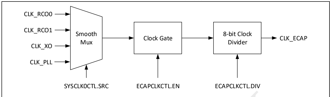
图 3-15: ECAP 时钟控制框图
