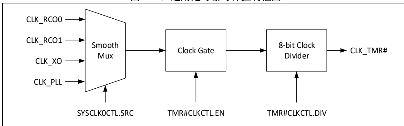
图 3-12：通用定时器时钟控制框图
