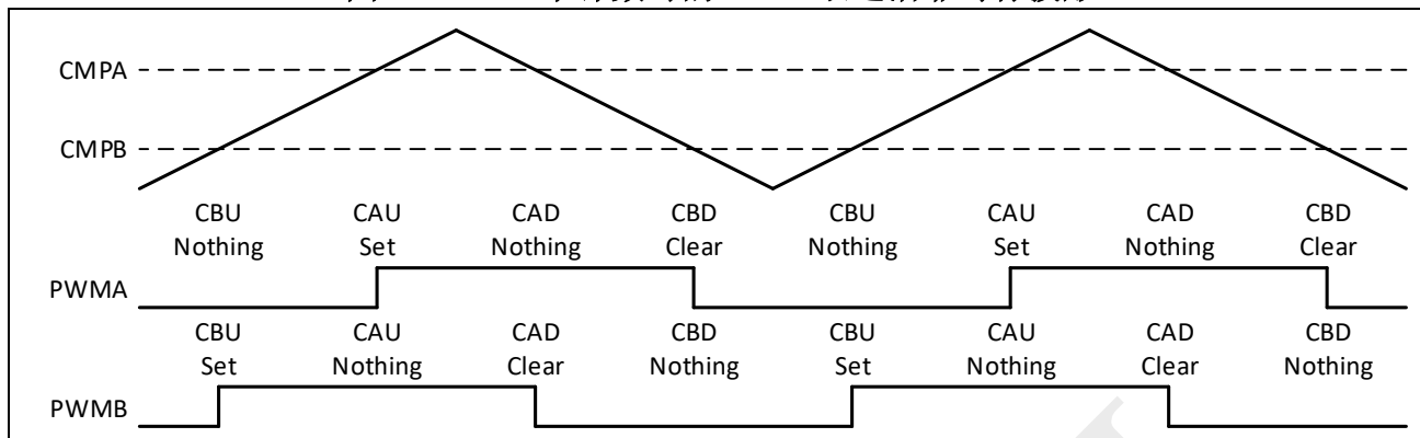
图 10-10: 上下计数时的 PWM 双边沿非对称波形
