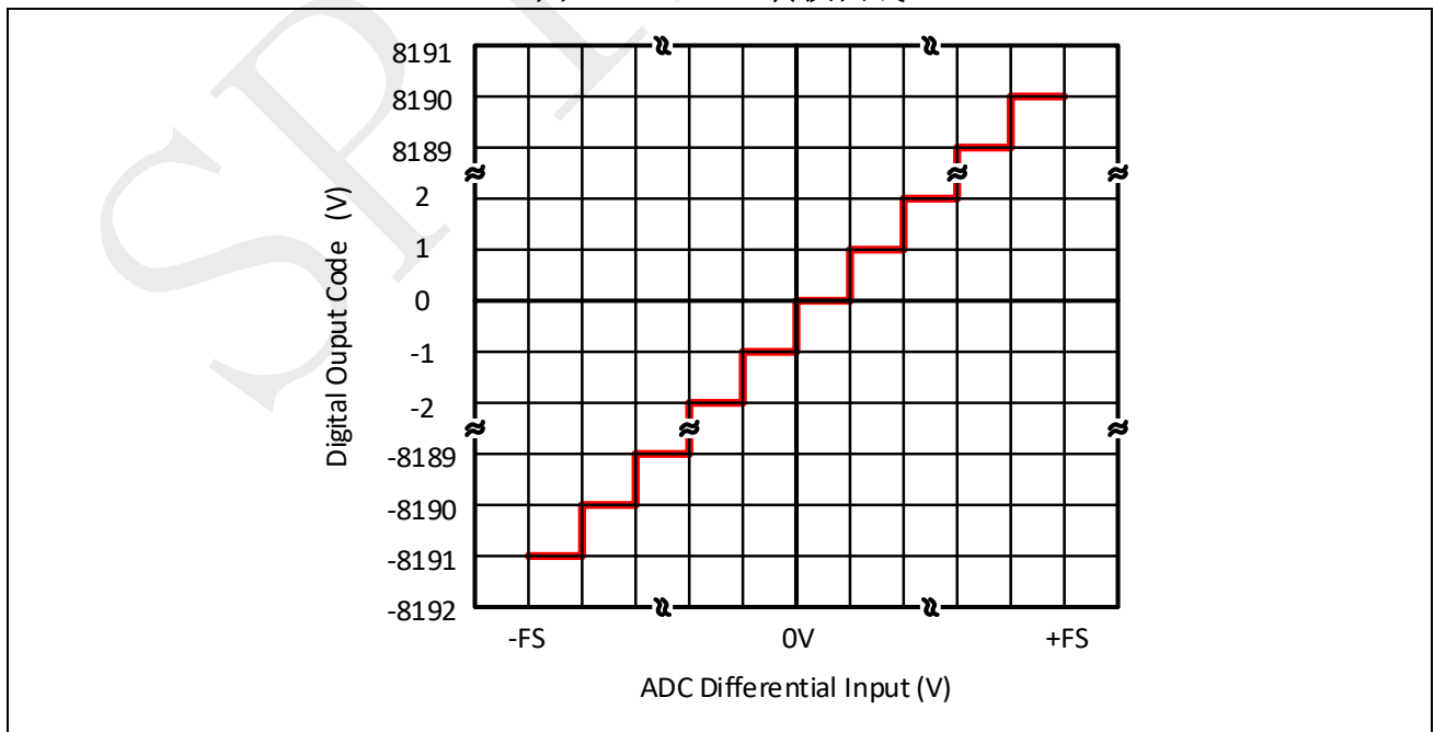
图 12-15: ADC 转换曲线
