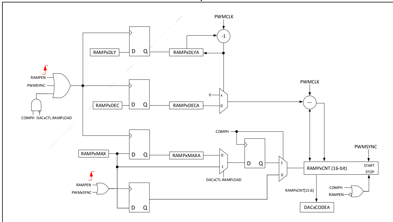
图 16-2: Ramp 发生器框图
