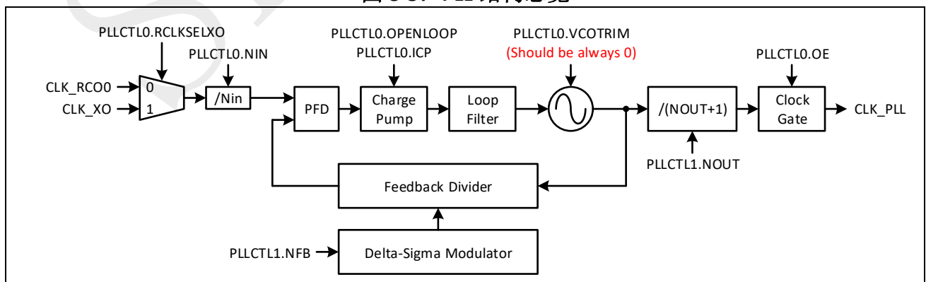
图 3-5: PLL 结构总览
