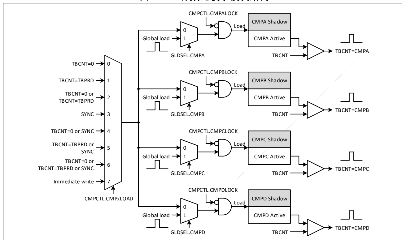
图 10-6：计数比较子模块结构
