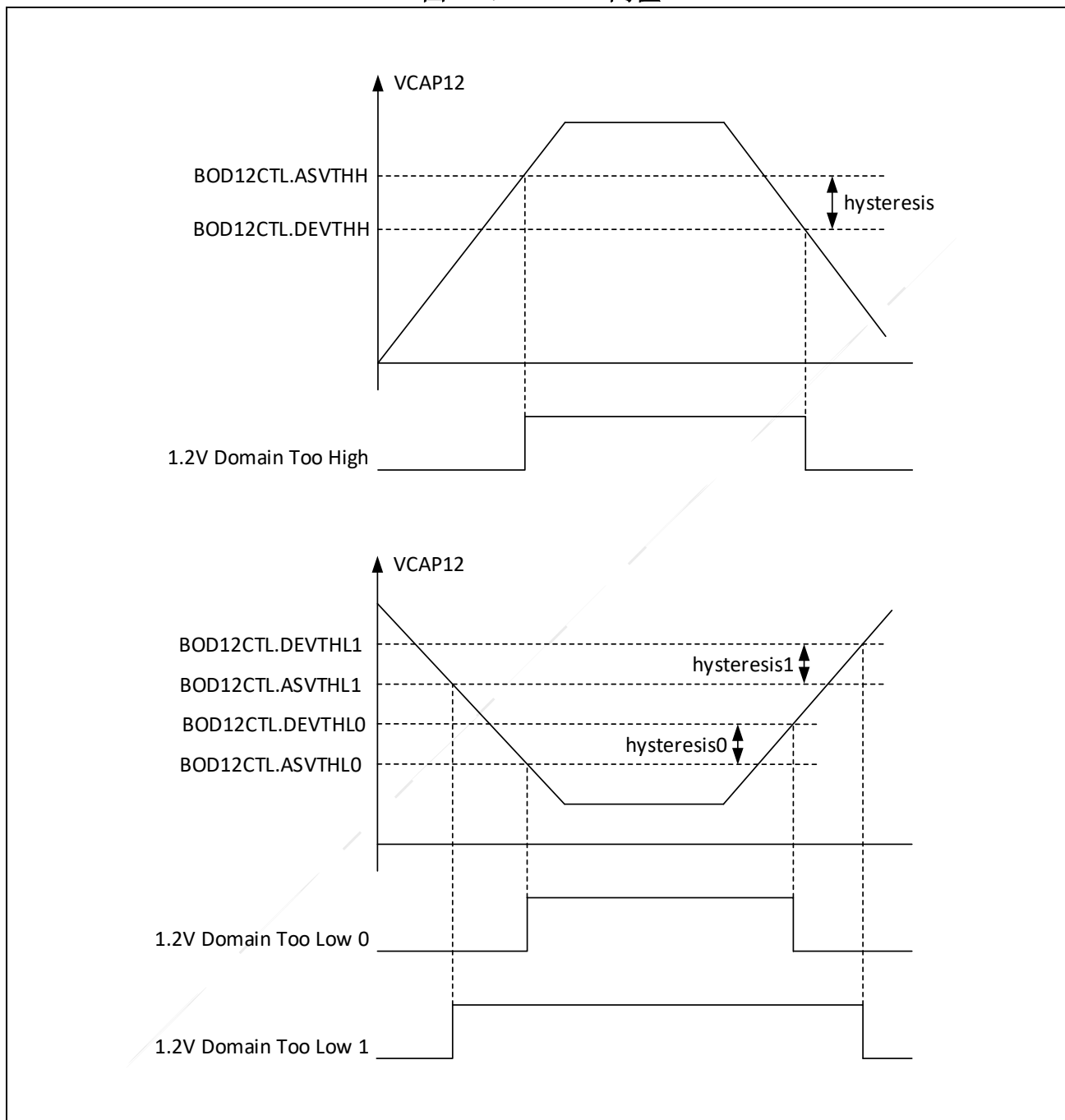
图 2-5: VCAP12 阈值
