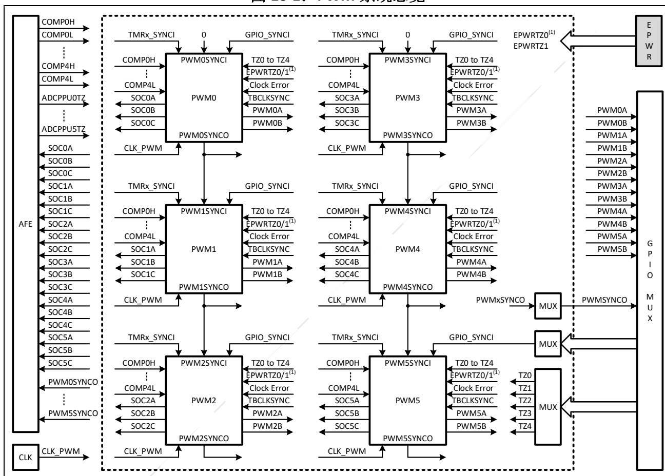
图 10-1: PWM 系统总览
