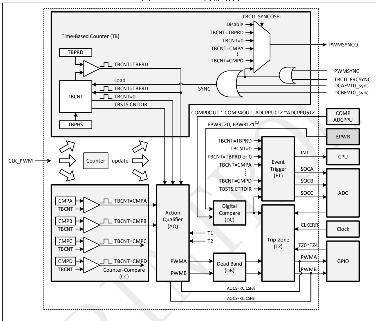
图 10-2: PWM 内部结构
