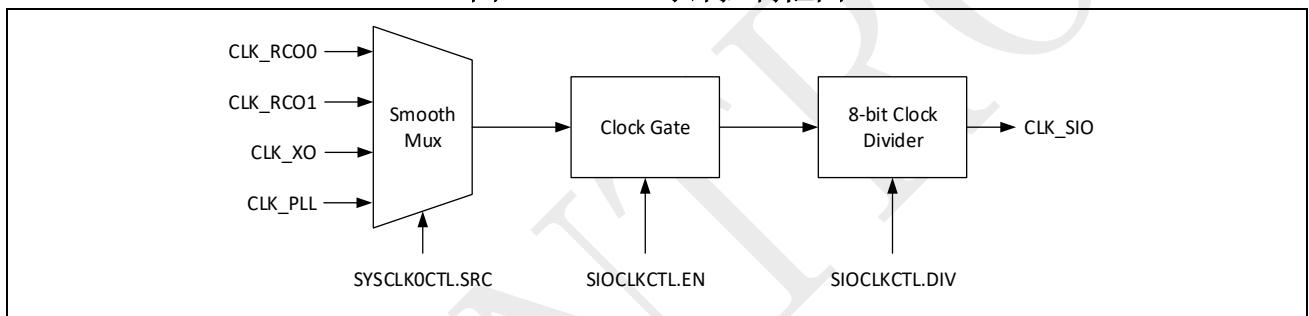
图 3-16: SIO 时钟控制框图
