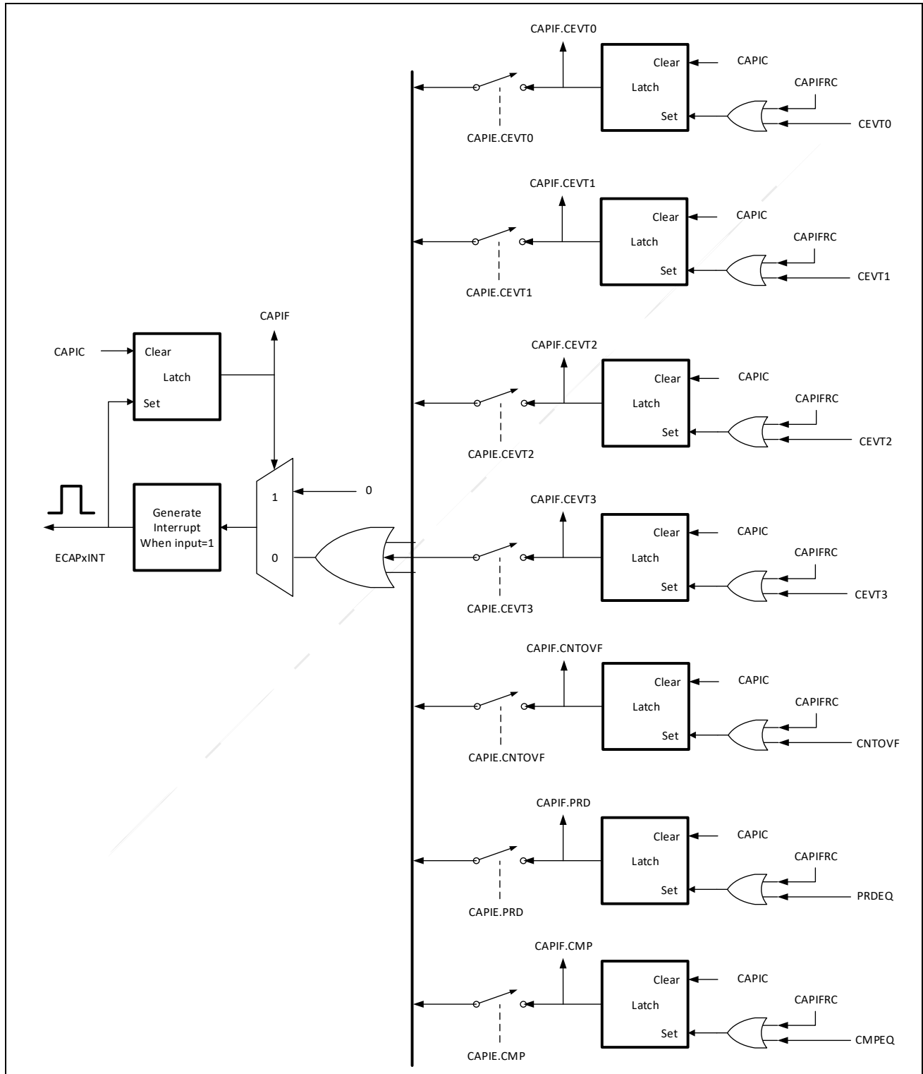
图 11-8: ECAP 模块的中断
