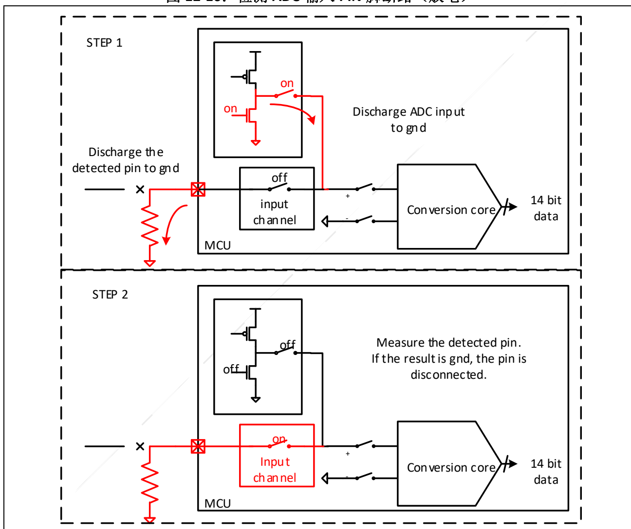
图 12-16: 检测 ADC 输入 PIN 脚断路（放电）
