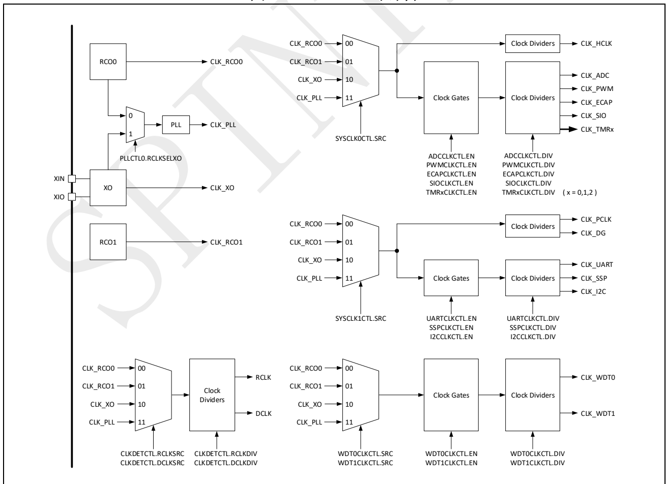
图 1-2: SPC1168 时钟树
