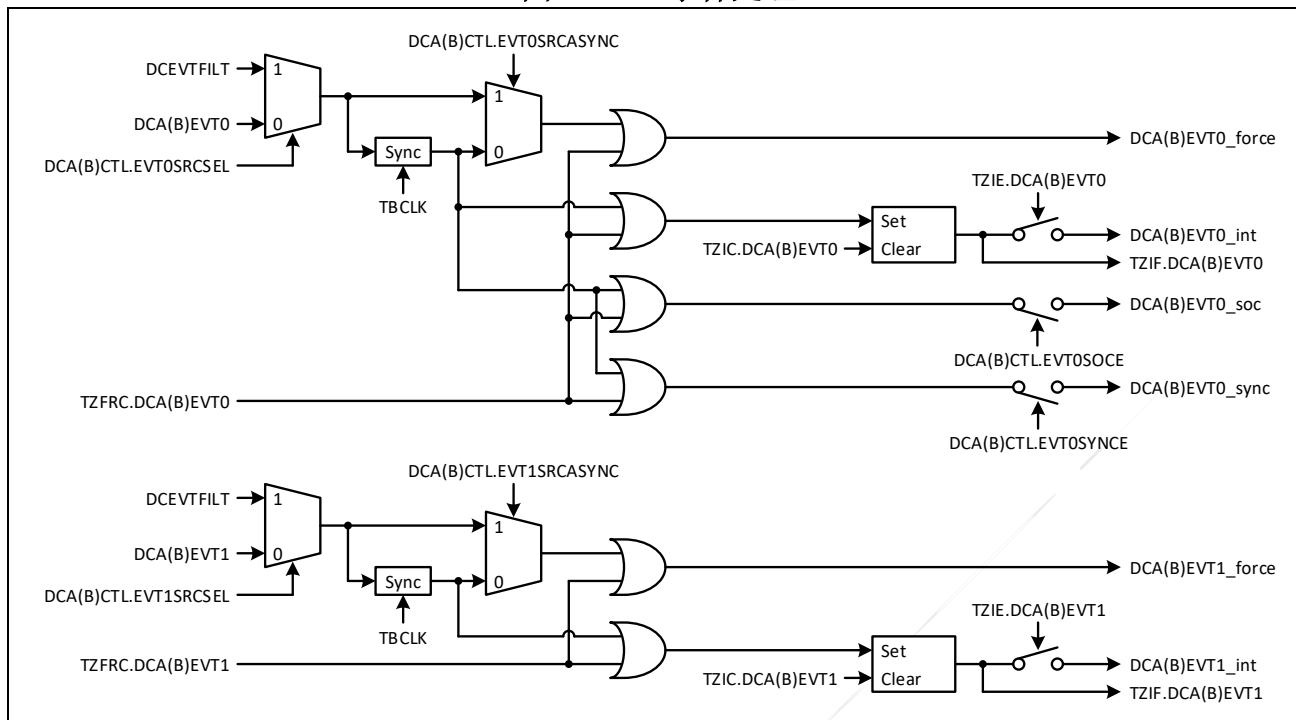
图 10-19: 事件处理
