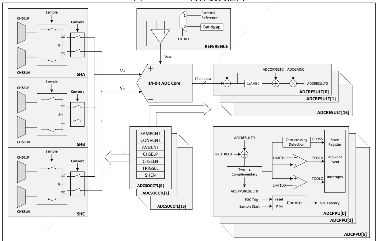
图 12-1: ADC 内部模块框图
