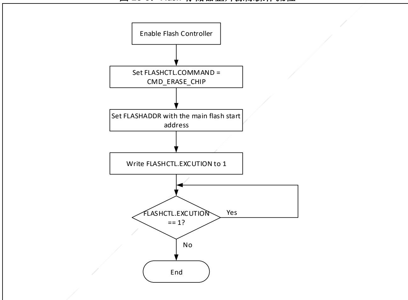
图 20-6: Flash 存储器整片擦除操作流程
