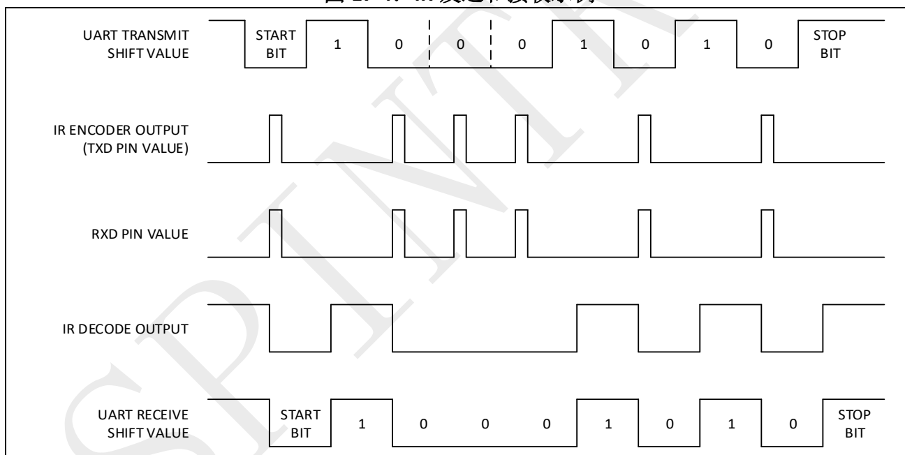
图 17-4：IR 发送和接收示例
