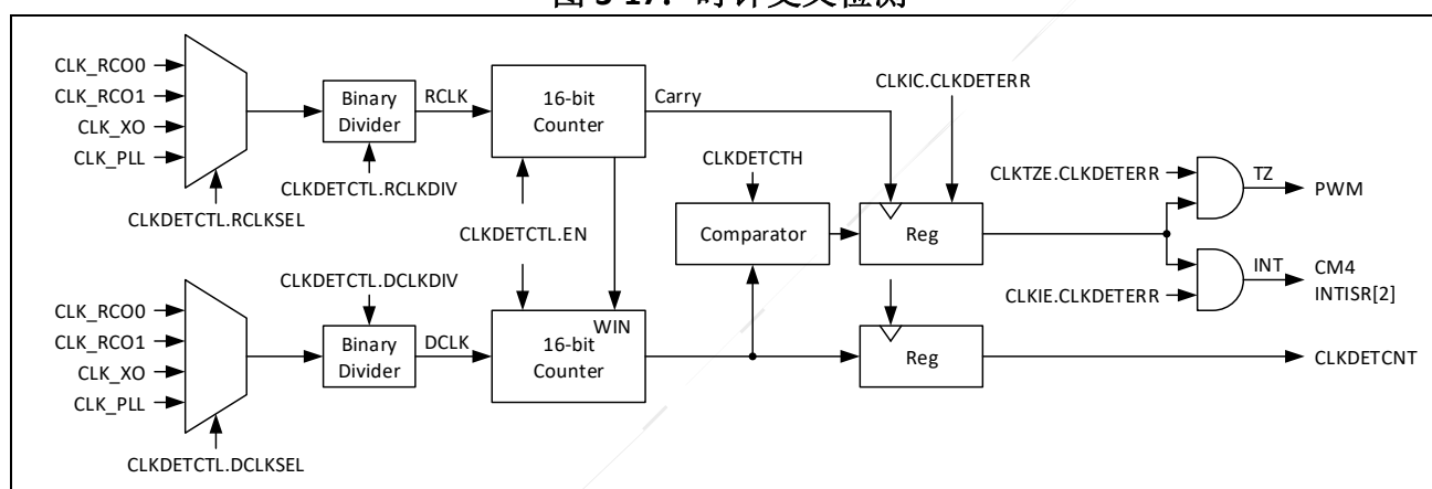
图 3-17：时钟交叉检测
