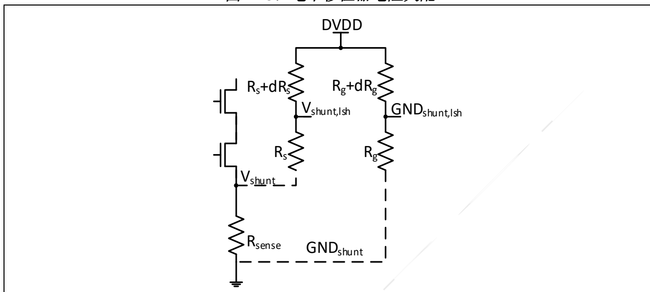
图 14-9：电平移位器电阻失配
