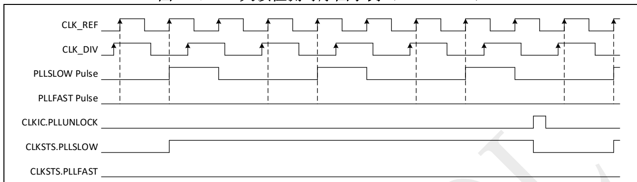
图 3-6: PLL 失锁检测时序图示例 ( F_{REF} > F_{DIV} )
